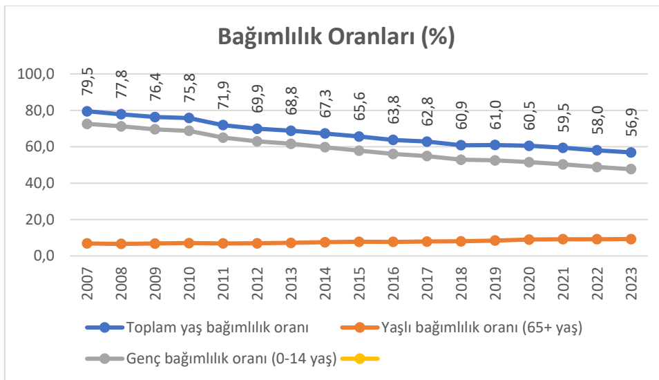
Şekil 5: Bağımlılık Oranları
